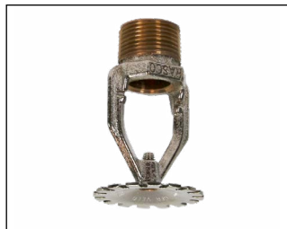
GFR VELO ECOH Pendant
