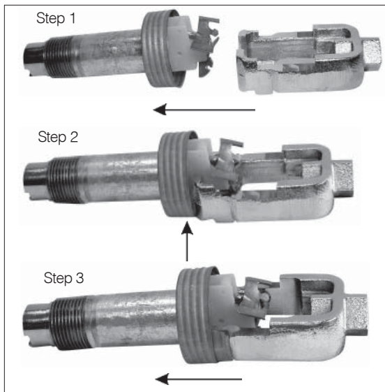
Fig. 2 - XLO2 Wrench
